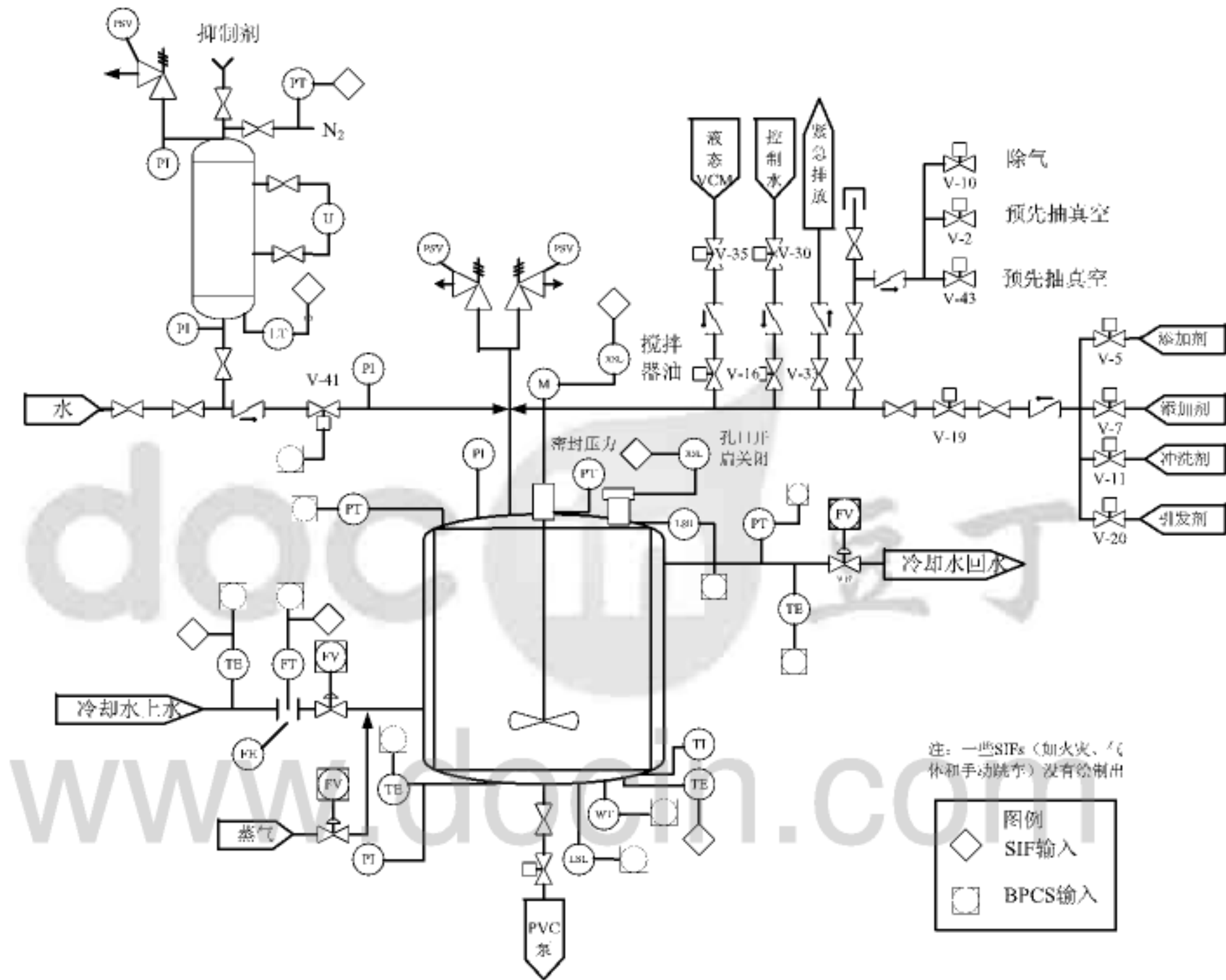
图 G.3 PVC 工艺简化 P&ID 图
