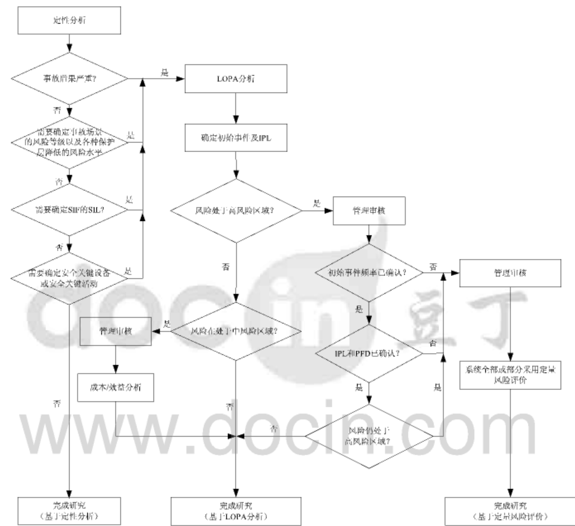
图 B.1 LOPA 的应用时机
