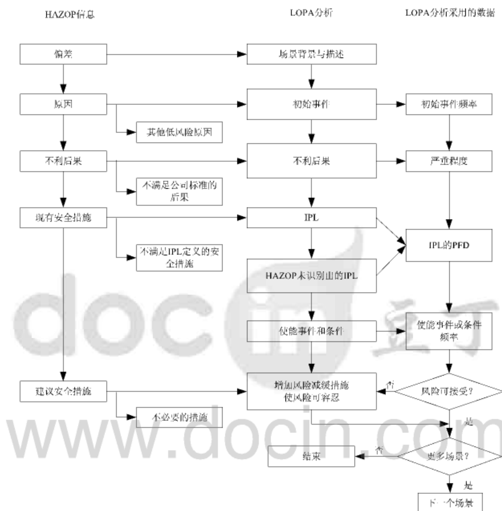
图 C.1 HAZOP 信息与 LOPA 信息的关系
