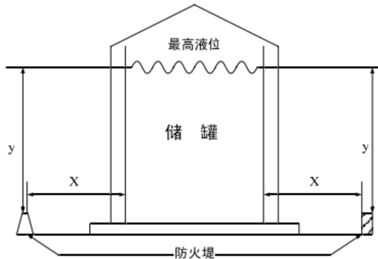
图 6.3.6 单防罐至防火堤内顶角线的距离
