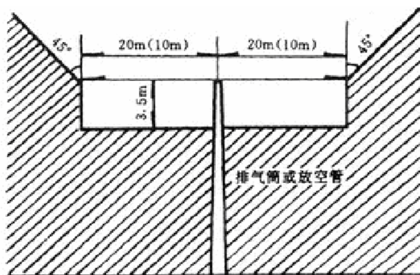
图 5.5.11 可燃气体排气筒、放空管高度示意图
